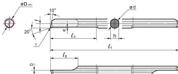
La figura mostra l'utensile con il romptrucioli.
